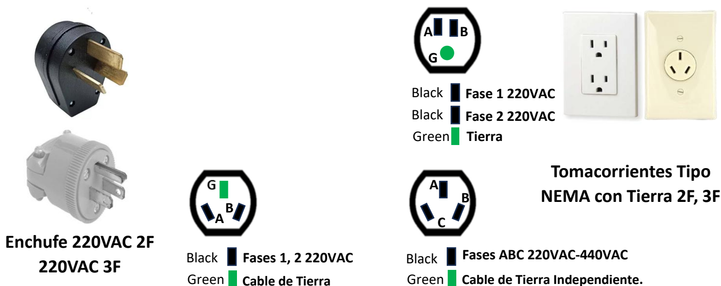
Figura # 2. Enchufe y Tomacorrientes Estándar con Tierra 220VAC 2F/3F.
