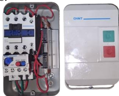
Figura # 5. Caja, Switch de Encendido y Apagado y detalle del Arrancador Directo 3F con Contactor.
